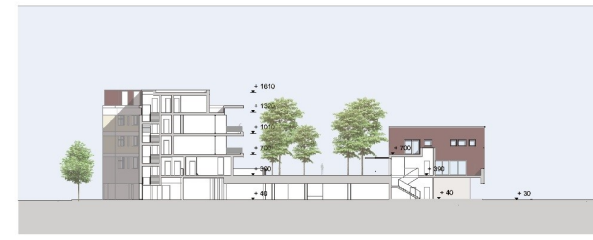
Sezione A-A
